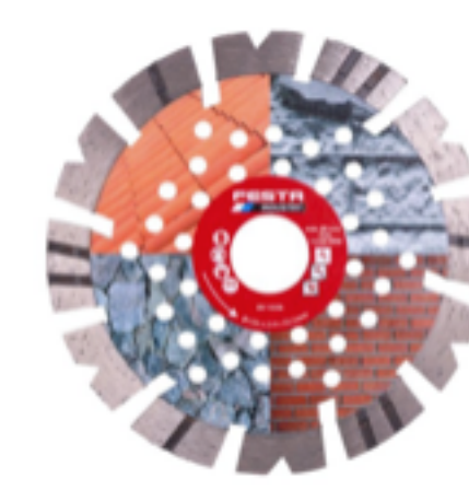
kód: 1996588 Kotúč diam. rezný segment. 125x2,4x22,2mm FESTA INDUSTRY 21240
